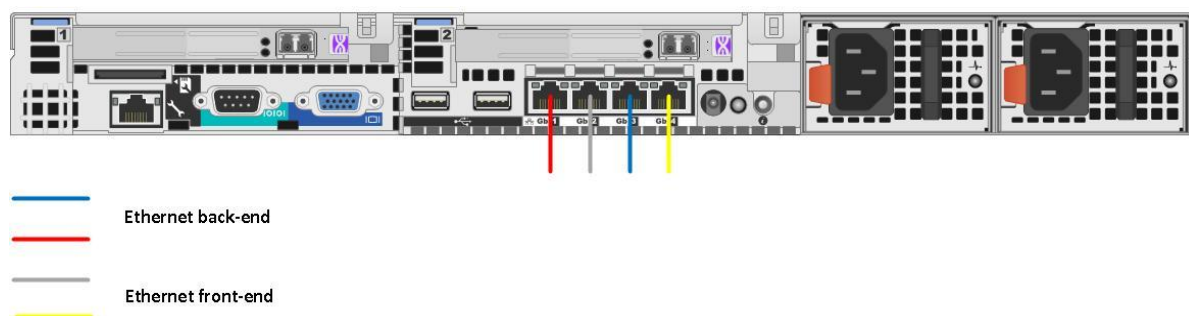
Rys. 56 - Porty węzła typu Back-end i Front-end
